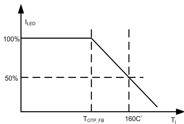
图 5: 温度反馈曲线
