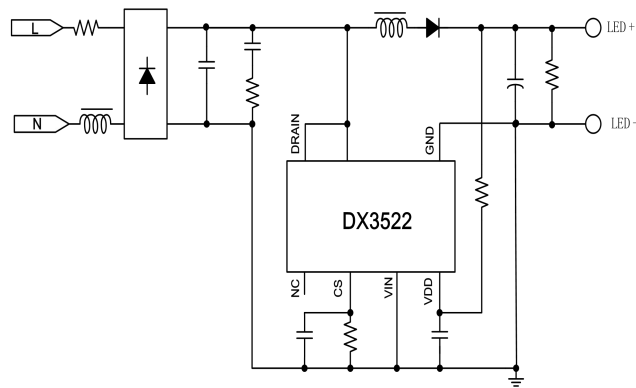
图 6: DX3522 BOOST 浮地结构
