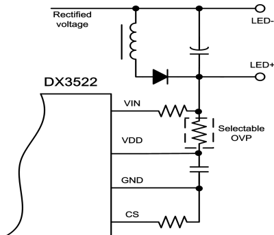
图 2: 共地结构 VDD 供电
