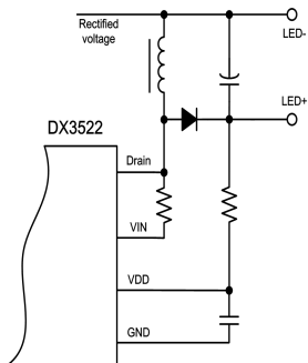
图4: LED开路时自锁保护线路
