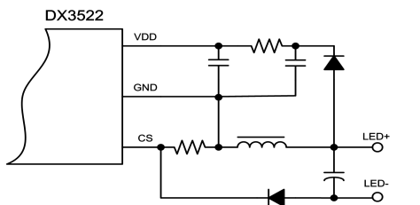
图 1:浮地结构 VDD 供电
